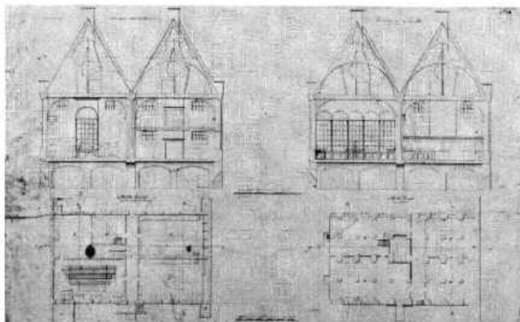
Dwarsdoorsneden en plattegronden, gemaakt voor de verbouwing van het hospitaal tot collegezaal, waarop de balkenconstructie en keldergewelven goed zichtbaar zijn, 1845. G.A.U. Top. Atlas Zk. 13.3 (1).
