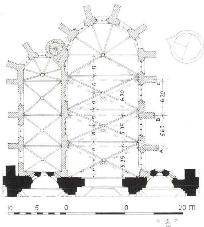
Afbeelding 2 Mariakerk, plattegrond van het gothische koor
