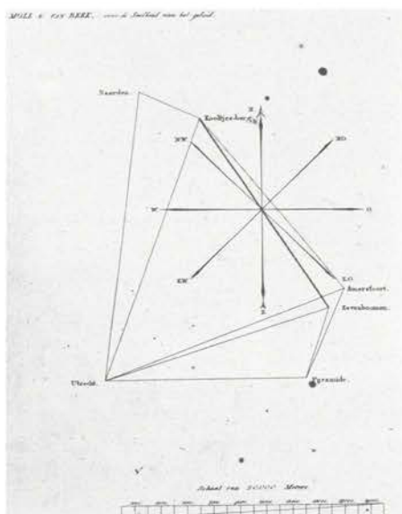
afb. 4: Situatie van het terrein bij de bepaling van de geluidssnelheid, waarop ook aangegeven staan de torens in Amersfoort, Naarden en Utrecht, benevens de pyramide te Zeist, welke gebruikt zijn bij de triangulatie, om de afstand Kooltjesberg en Zevenboomen nauwkeurig te kunnen berekenen. (foto: J. P. Stolp, Utr. Universiteitsmuseum).
