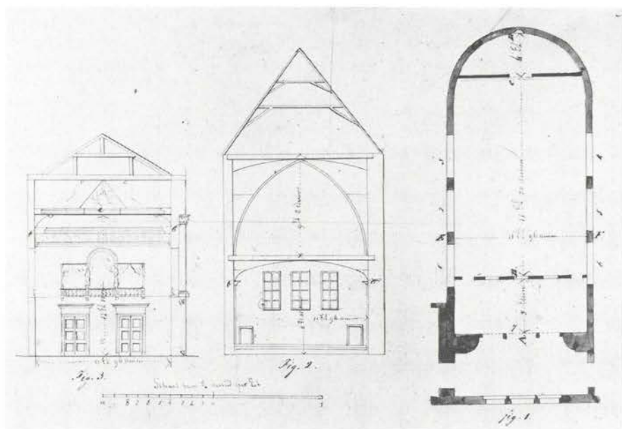
8. J. van Maurik, Doorsnede en plattegrond van de concertzaal, 1840. Links de geprojecteerde verbouwing, in het midden de bestaande situatie en rechts de bestaande situatie met de geprojecteerde veranderingen. BC geeft de lengte van de zaal in de bestaande situatie aan, AD die van de oorspronkelijke lengte van het koor. G.A.U., IV, 1004++
