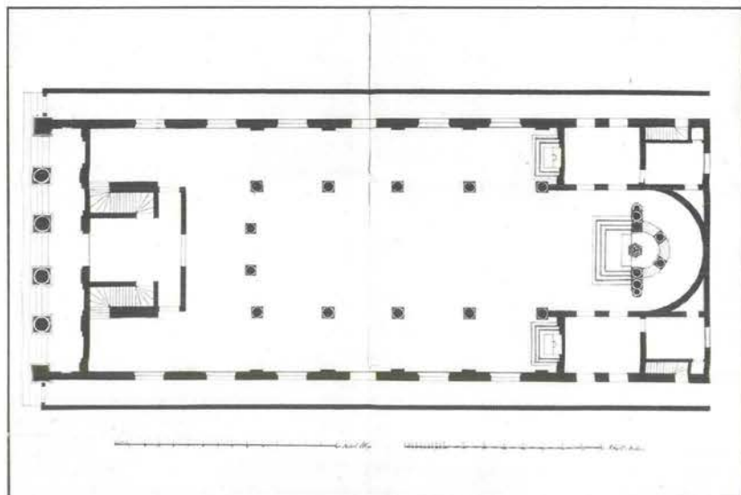
St. Augustinus, 1e ontwerp, 1837, grondplan, in: ARA, RKE 482: 30-6-1837 no. 1471/7. Foto ARA.
