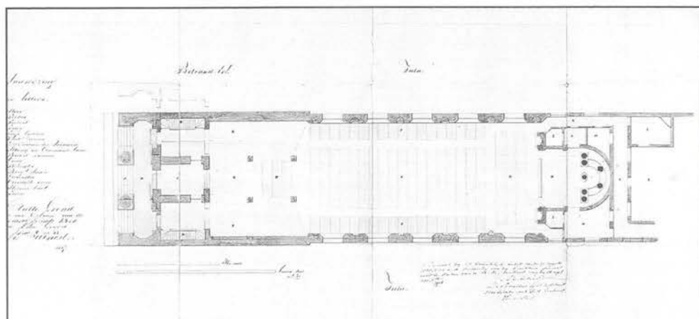
St. Augustinus, 2e ontwerp, door K.G. Zocher, 1837, plattegrond. ARA, Top. Atlas, RK-ARA-2e Afd.-1838-3 GF 88377. Foto ARA.
