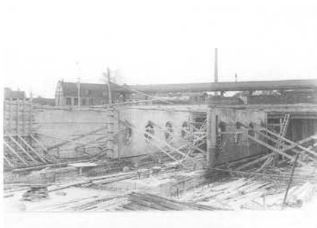
Rechts: Eerste (westelijke) deel Leidseveertunnel in aanbouw, 1937. De keermuren, steunmuren en tunnelvloer zijn gereed; op de achtergrond de perronkap van het Buurtstation. Foto Verz. NVBS.
