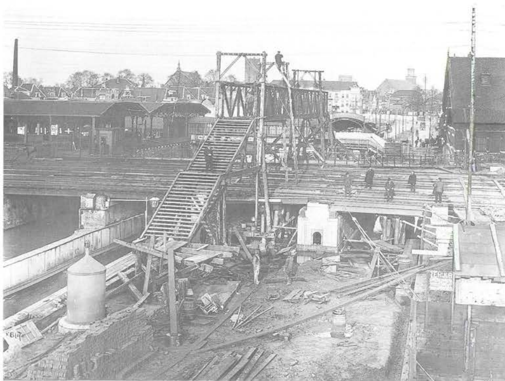
Onderdoorgangen in de Leidseweg in aanleg, gezien in de richting van de stad, 1907. Geheel links het Buurtstation en de doorgang voor rijverkeer, in het midden de tijdelijke voetgangersbrug, hier al buiten dienst, daarnaast de nieuwe onderdoorgang voor langzaam verkeer. Rechts het MESS / NCS station waarvan alleen het postgebouw te zien is. Foto Verz. J.G.C. van de Meene.
