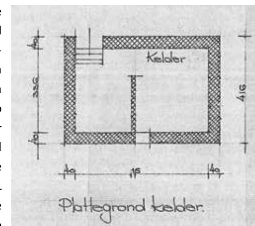
Plattegrond van de kelder van Het Spijk met daarin de lengte- en breedtemaat en de muurdikte. Tekening arch. bureau Jonkman en Van Dorp uit Zeist 1962. Collectie Regionaal Archief Zuid-Utrecht, archiefnr. 415, inv.nr. 1202.
