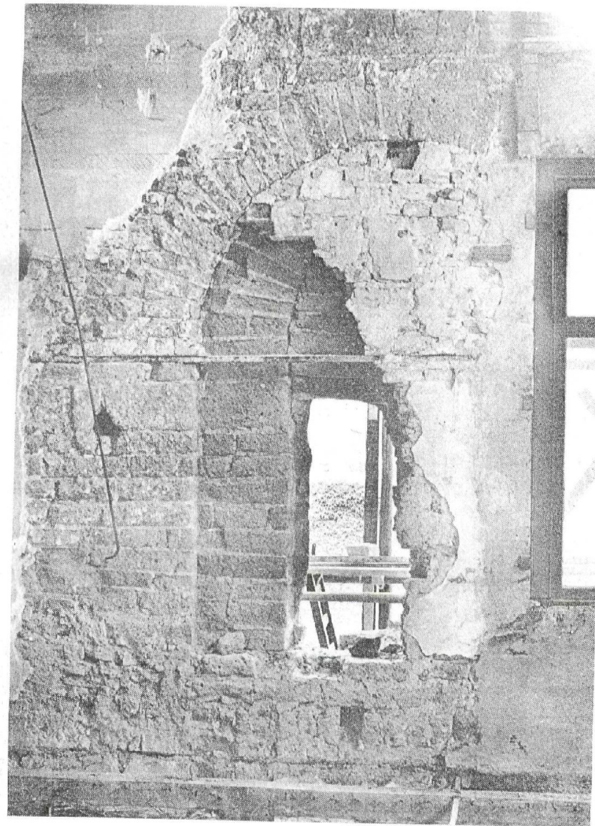
Westelijk venster in de zuidelijke transeptgevel (binnenzijde) van de Sint Paulusabdij komt tevoorschijn. Dit venster vindt men op het schetsplan terug en wel aan de buitenzijde rechts.
