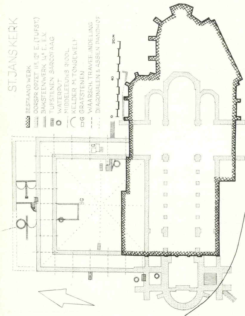
Afb. 1. Plattegrond van de St. Janskerk en de pandhof in hun oorspronkelijke gedaante volgens gegevens, afkomstig van onderzoeken door de Rijksdienst voor de Monumentenzorg, de Rijksdienst voor het Oudheidkundig Bodemonderzoek en de Dienst van Openbare Werken te Utrecht.
