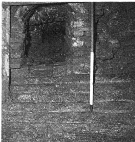
Afb 13. Van Asch van Wijckskade. Uitgang van het riool uit 1545.
