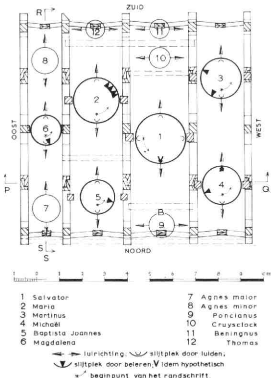
plattegrond van de klokkenstoel ter hoogte van T-U met de plaatsen van de klokken
