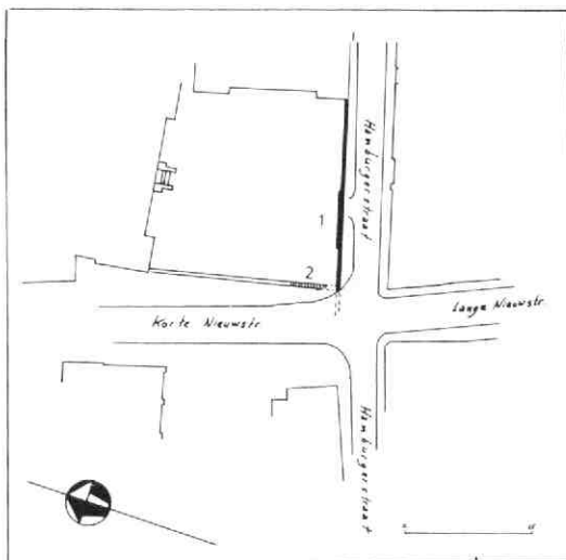
Afb 22. Hamburgerstraat 28. Situatie van de zuidelijke immunitetsmuur van de Paulusabdij en van de restanten van de bebouwing langs de oostzijde van de Korte Nieuwstraat. Opm. L. van Geffen. Tek. T. J. Hoekstra.
