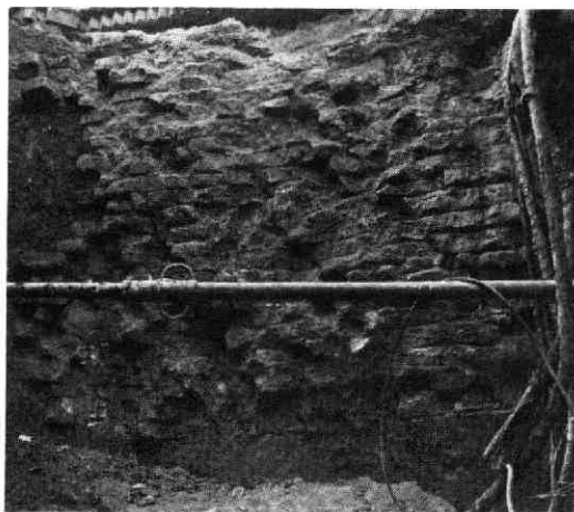
Afb 37. Lange Smeestraat. Resten van de Smeeteren (?). Het is niet duidelijk of links boven sprake is van een insteek voor de toren of van een sloperssleuf.
