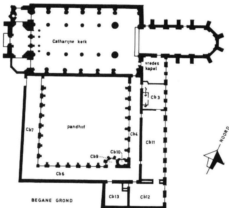
Afb 31. Lange Nieuwstraat, Catharijne Convent. Plattegrond op begane grond niveau. De Karmelieten bouwden de delen Cb 11, Cb 12 (het hoofgebouw; de dubbele muur is een toevoeging van de restauratie), Cb 13 (keukengebouw) en de delen van Cb 4 en Cb 6 (kloostergangen) tot aan de grenzen van resp. Cb 11 en Cb 13. Hoever ze met de kerk kwamen is onduidelijk. In de eerste fase vlak na 1529 hebben de Johannieters Cb 6 en 7 en de kerk afgemaakt. Na 1561 is de aansluiting met de kerk (Cb 3, Vredeskapel en een deel van Cb 4) gevolgd. Aan de aanleg van een kloostergang langs de kerkwand komen ze niet meer toe. Het meest westelijke deel van de kerk is van 1901. Tek. C. J. W. J. Hoeflaken.
