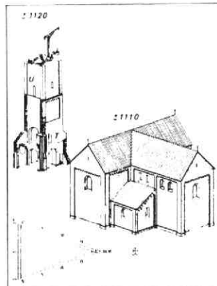
Opengewerkte scheve projectie: toestand 1100-1120. U: thans niet gebruikte deur met keperboog.
