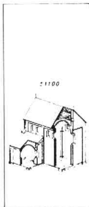
Opengewerkte scheve projectie: toestand 1100-1120. U: thans niet gebruikte deur met keperboog.
