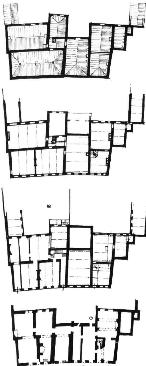
Afb. 20 Donkerstraat 15-19. Reconstructie-schets van de plattegronden van het huis Zoudenbalch. Tek. A. F. E. Kipp.
