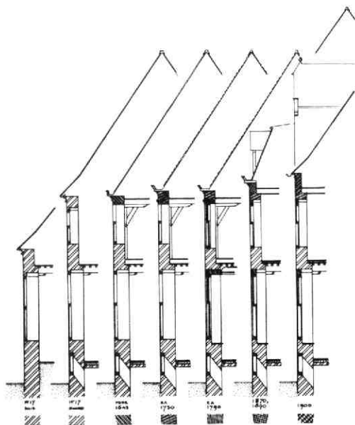
Afb. 51 Janskerkhof 3. Evolutie van de Statenkamer in doorsnede (oostmuur) en gevelaanzicht. Iedere travée vertegenwoordigt een nieuwe fase. Tek. A. F. E. Kipp.
