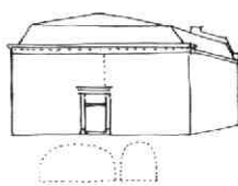
Afb. 55 Kromme Nieuwe Gracht 56. Schets van de ontwikkeling van het huis. Tek. A. F. E. Kipp. 1: middeleeuwse situatie. 2: 17e en 18e eeuw. 3: verbouwing van ca. 1860.
