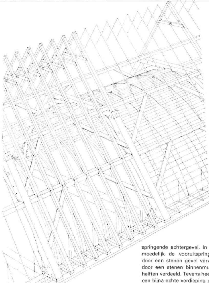
Afb. 57 Lange Smeestraat 40. Isometrie van de middeleeuwse kap en houten tongewelf van de noordvleugel van het Bartholomeïgasthuis. Tek. K. Rampart.
