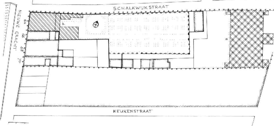
Afb. 98 Schalkwijkstraat 11. Situatie met de reconstructie van de oorspronkelijke opzet van de slangenmuur ca. 1732. Tek. A. F. E. Kipp. a: Leeuwenberchgasthuis. b: Nieuwe Gracht 64.
