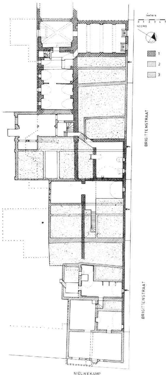
Afb. 15 Brigittenstraat 1-9. Plattegrond op kelderniveau. Tek. E. M. Kylstra en A. F. E. Kipp. 1: middel-eeuws muurwerk. 2: 17e eeuws. 3: 19e eeuws. 4: achtergevelgrens volgens de kadastrale minuut van 1821.
