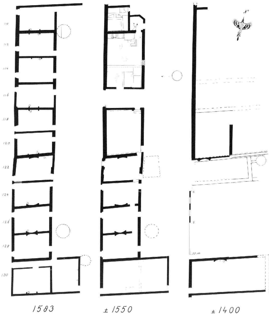
Afb. 102 Springweg 130-130bis. Overzicht van de drie fasen van de bebouwing ter plaatse van de Mieropskamen in ca. 1400, ca. 1550 en 1583. De kleine cirkeltjes bij de stookplaatsen geven de haardpotten aan. Tek. B. J. M. Klück.
