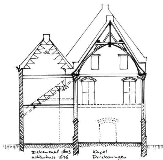
Afb. 13 Brigittenstraat 1-9. Doorsnede naar het westen van Brigittenstraat 5 door de voormalige Driekoningenkapel (rechts) met de in 1603 aangebouwde ziekenzaal en het achterhuis uit 1636 (links). Tek. A. F. E. Kipp.
