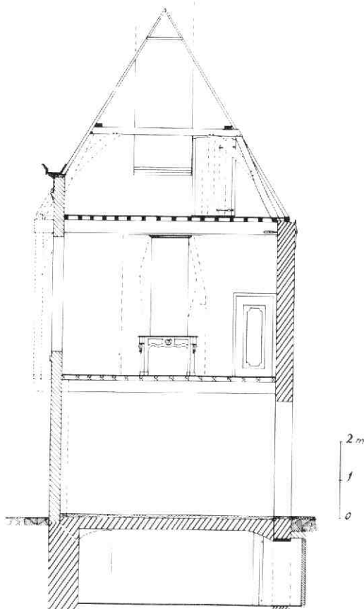
Afb. 76 Mariaplaats 9. Doorsnede naar het noorden. Tek. B. J. M. Klück, E. M. Kylstra. De bewaard gebleven onderdelen van de middeleeuwse kap zijn met getrokken lijnen aangegeven. Het verdwenen gedeelte is gestippeld. Dat geldt ook voor de constructie die bij de oorspronkelijke overkragende gevel hoort. De maten daarvan volgen uit het aanvullen in de opmeting van de verdwenen onderdelen van de kap. Tevens valt de mate van overkraging af te leiden uit de afwijking van het wapenschild op de zuidmuur ten opzichte van het hart van de muur.
