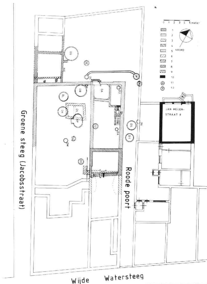
Afb. 34 Jan Meijenstraat e.o. Overzichtsteekening van de gevonden bouwingsresten, aangevuld met behulp van de kadastrale minuut van ca. 1821 en verbouwings-tekeningen uit het begin van de 20e eeuw. Tek. A. M. Kylstra.
