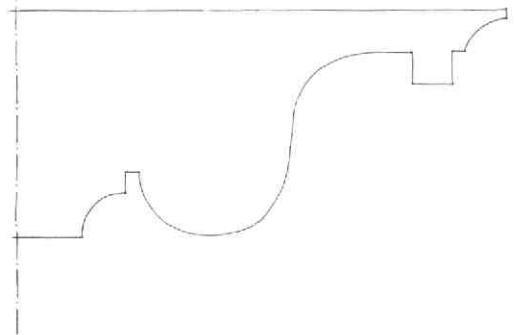
Afb. 80 (Lange) Minderbroederstraat 1 en Korte Minderbroederstraat 23. Sleutelstuk van de rechter strijk balk op de eerste verdieping van nr 1. Tek. A.F.E. Kipp.
