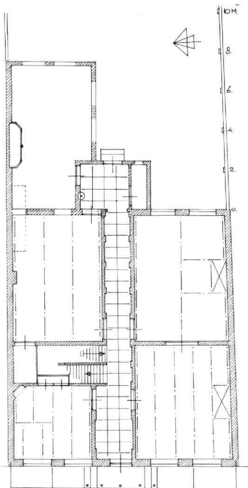
Afb. 17 Boothstraat 17. Reconstructie van de plattegrond van beganegrond en verdieping na de 18e-eeuwse verbouwing. Tek. A.F.E. Kipp.
