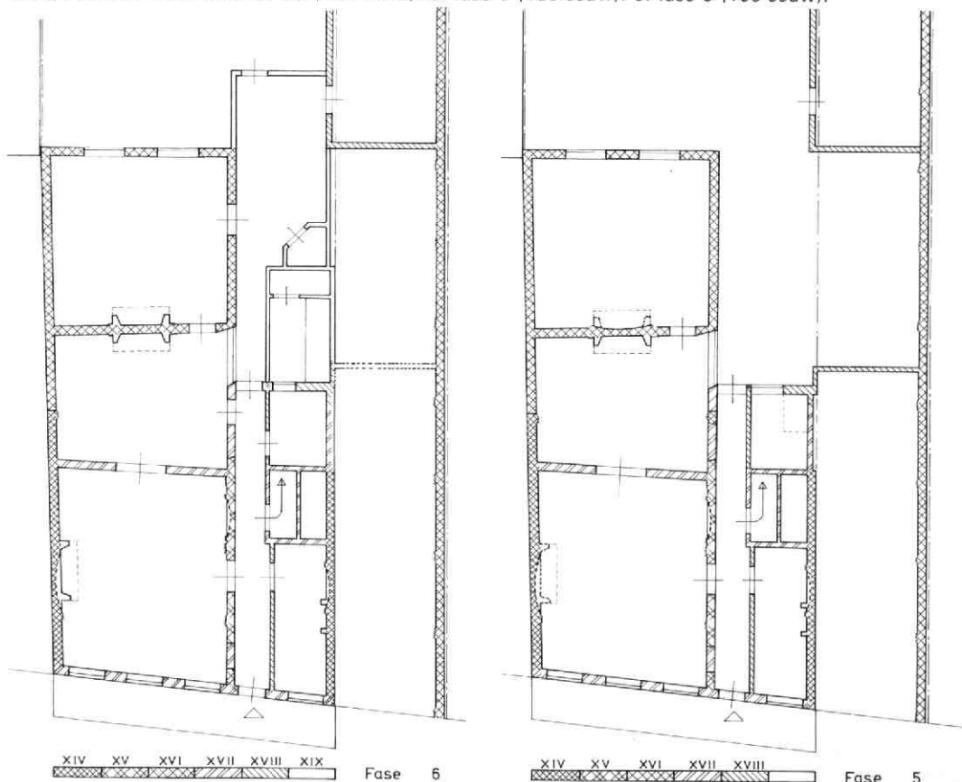
Afb. 100 Nieuwe Gracht 68. De ontwikkelingsstadia van het huis, weergegeven in de plattegrond van de be- ganegrond. Tek. Kees Terhorst en A.F.E. Kipp. 1: fase I (14e eeuw?). 2: fase IIa en IIb (15e eeuw). 3: fase III (16e eeuw). 4: fase IVa en IVb (17e eeuw). 5: fase V (18e eeuw). 6: fase 6 (19e eeuw).
