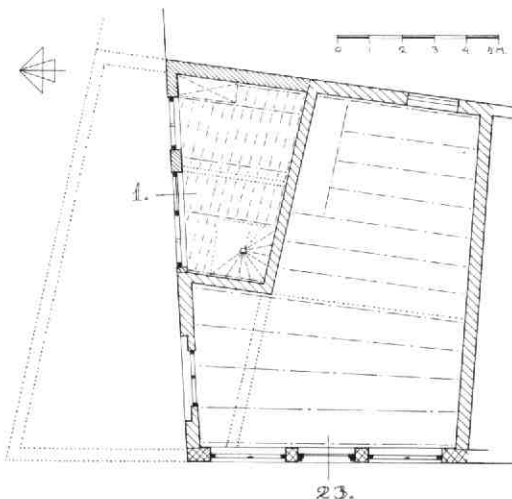
Afb. 79 (Lange) Minderbroederstraat 1 en Korte Minderbroederstraat 23. Schematische plattegrond van de begane grond van de beide huizen, met aanduiding van de middeleeuwse voorgangers. Tek. A.F.E. Kipp.
