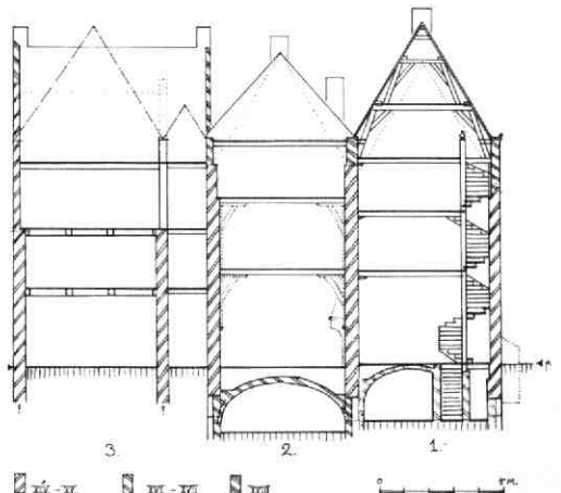
Afb. 85 Neude 1 en 2. Reconstructie van de dwarsdoorsnede door de huizen Neude 1, 2 en 3, naar achteren gezien. Tek. A.F.E. Kipp. a: toestand in de 15e eeuw. b: toestand na de 17e-eeuwse verbouwingen.
