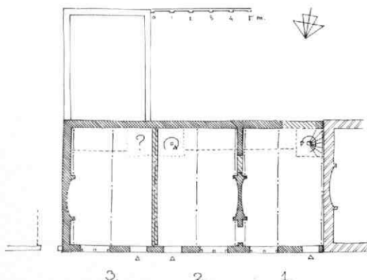
Afb. 12 1e Achterstraat 2 en 3. Plattegrond van de beganegrond van het huis, met bouwsporen. Tek. A.F.E. Kipp.
