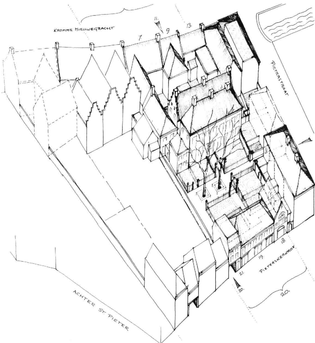
Afb. 139 Pieterskerkhof 20. Vogelvlucht-reconstructieschets van de bebouwing op het claustrale erf van Pieterskerkhof 20 en Kromme Nieuwe Gracht 7-13, en op het aangrenzende erf (Kromme Nieuwe Gracht 1-5), gezien vanuit het zuidwesten; toestand vóór 1925. Tek. A.F.E. Kipp.
