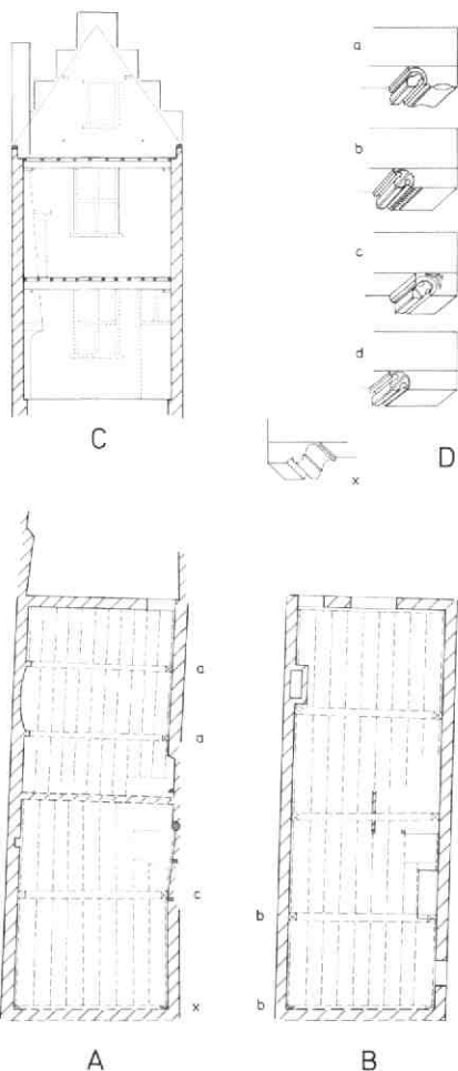
Afb. 93 Nieuwe Gracht 53 en 55. Plattegronden met de aangetroffen bouwsporen en balklagen. Tek. Kees Terhorst. A: de begane grond. B: de verdieping. C: reconstructie: doorsnede naar de achtergevel gezien. D: de verschillende typen sleutelstukken.
