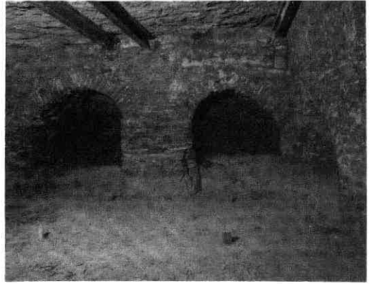
Afb. 84 Neude 1 en 2. Foto van de fundering op spaarbogen onder het voorste deel van nr 1, gezien naar voren, na de ontgraving.
