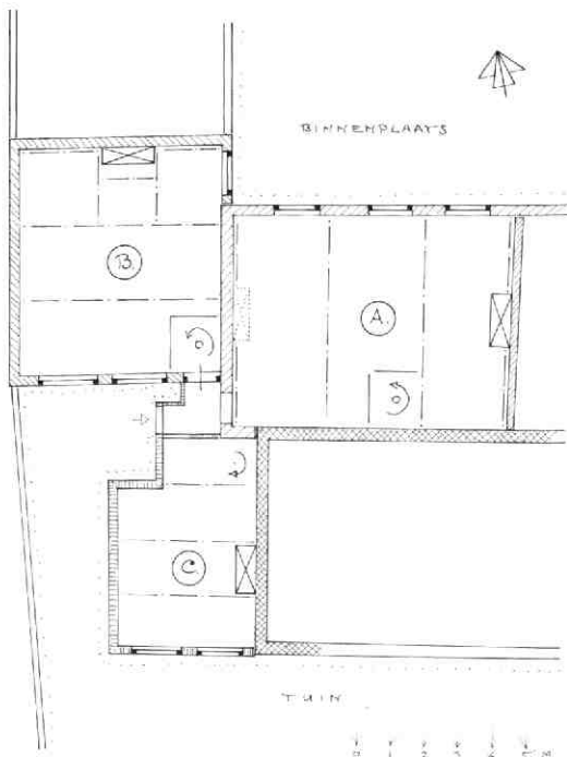
Afb. 138 Pieterskerkhof 20. Plattegrondscheets van de beganegrand van de tijdens de laatste verbouwing onderzochte delen van het complex. Tek. A.F.E. Kipp. A: het westelijke deel van de achterbeuk van het hoofdhuis. B: het achterste zijhuis. C: het voorste zijhuis.
