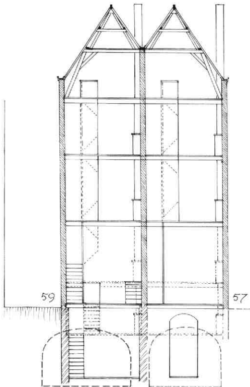
Afb. 96 Nieuwe Gracht 59. Principeddoorsnede door het 18e-eeuwse dubbelhuis. Tek. A.F.E. Kipp.
