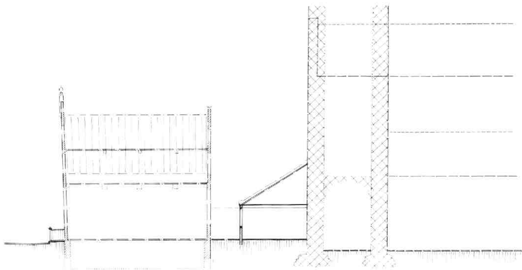
Afb. 71 Korte Nieuwstraat 6. Langsdoorsnede door het huis, naar het noorden gezien. Boven: de 17e-eeuwse opzet. Tek. A.F.E. Kipp. Onder: de huidige toestand. Tek. J.J. Jeehee en A. Warffemius (RDMZ), bewerkt en aangevuld door A.F.E. Kipp. Links het voorhuis, rechts het achterhuis met aanduiding van de verschillende groeifasen en gestippeld het westfront van de romaanse Pauluskerk, waar het oudste achterhuis tegen-aangebouwd was.
