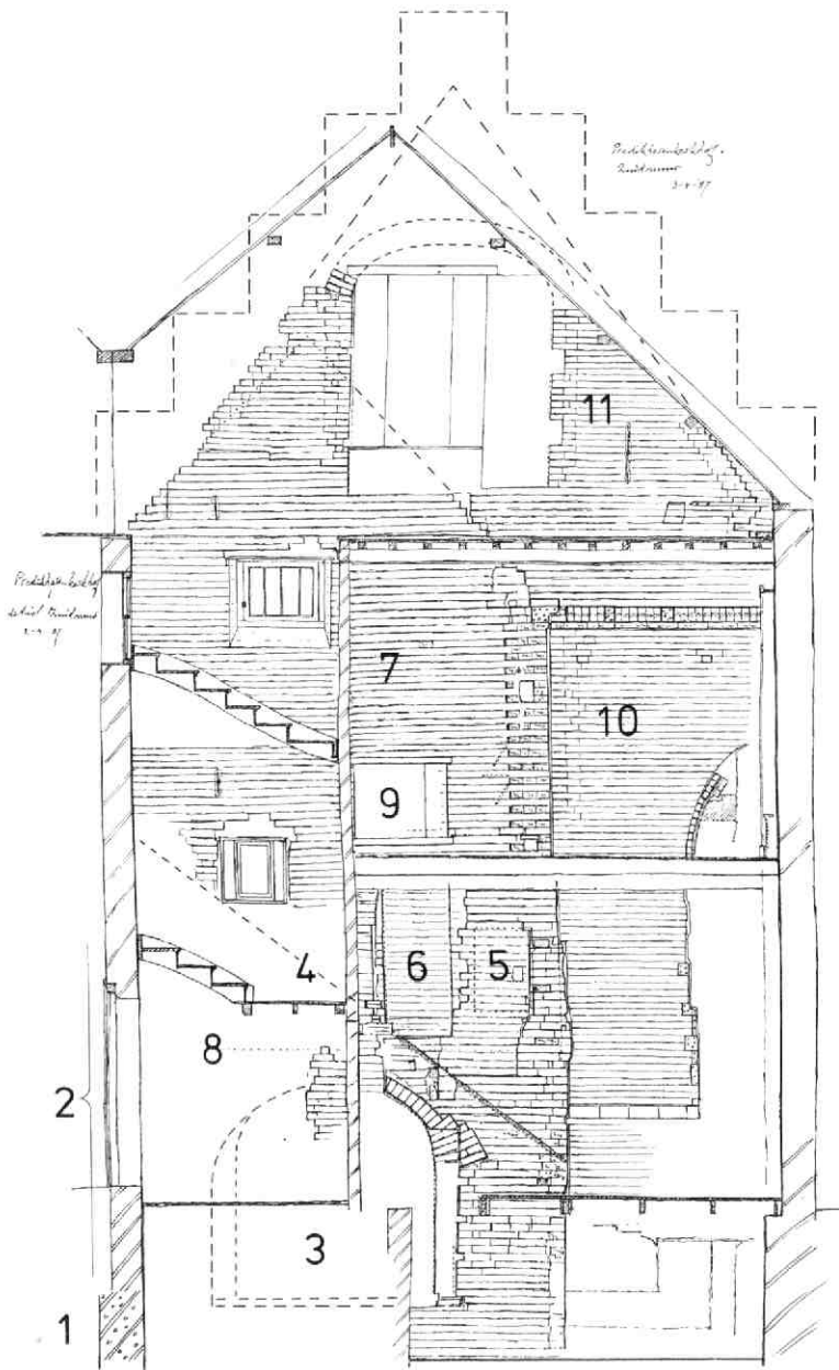
Afb. 148 Predikherenkerkhof 1. Bouwsporen in de zuidmuur van het voorhuis. Tek. Bart Klück. 1: tufstenen fundering. 2: muurwerk (midden 13e eeuw). 3: (later versmalde) rondboog-opening. 4: daklijn. 5: luikopening, later verplaatst naar 6. 7: gevel van de 14e-eeuwse verhoging. 8: 14e-eeuwse vloerlijn met doorgang ter plaatse van 6. 9: venstertje (ca 1500). 10: muurfragment (ca 1500) met spitsboogvenster en doorgehakte daklijst. 11: gevel van na 1554.
