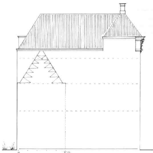
Afb. 28 Breidstraat 4. Schets van de westelijke zijmuur, met de topgevel van het oorspronkelijke achterhuis. Tek. A.F.E. Kipp.
