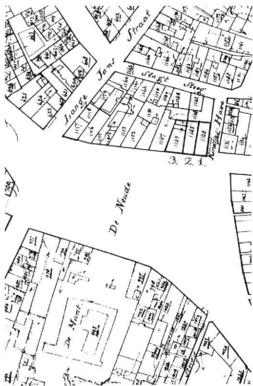
Afb. 81 Neude 1 en 2. Situatietekening op basis van de kadastrale minuut van 1832. Tek. A.F.E. Kipp.
