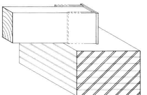
Afb. 125 Oude Gracht 151. De oplegging van de 13e-eeuwse dennebalken met de afscherming door middel van eiken plankjes. Tek. Jan van der Hoeve.
