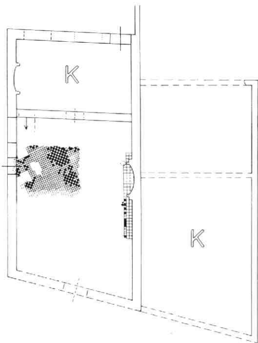
Afb. 161 Springweg 67. Plattegrond van nr 67 (rechts) en nrs 69-71 met hun indeling. K = onderkelderd. Tek. Bart Klück en Kees Terhorst.
