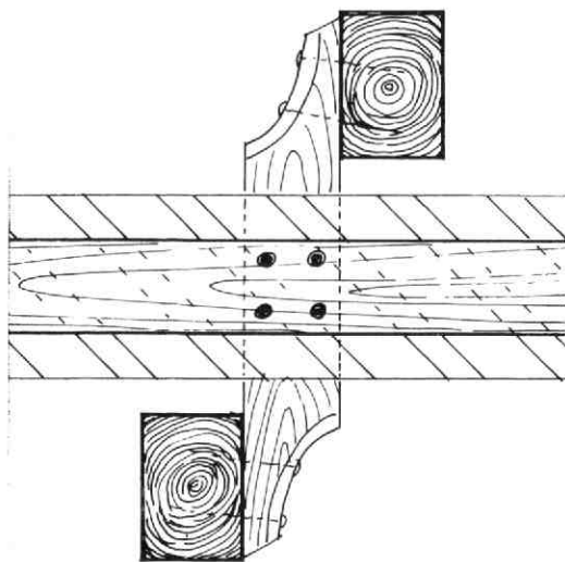
Afb. 25 Boothstraat 17. Bovenaanzicht van de blokkeels in de middenmuur op zolder. Tek. A.F.E. Kipp.
