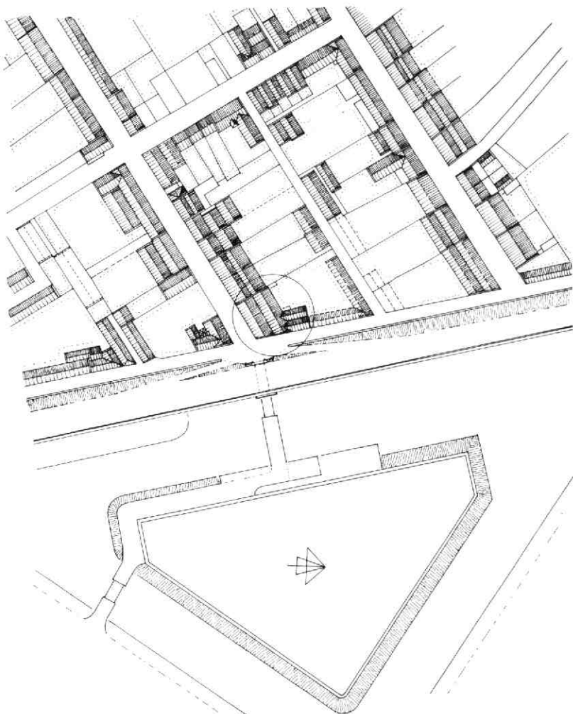
Afb. 74 Lepenburg 1. Situatietekening met kappenplan van de toestand in de tweede helft van de 17e eeuw. Tek. A.F.E. Kipp.
