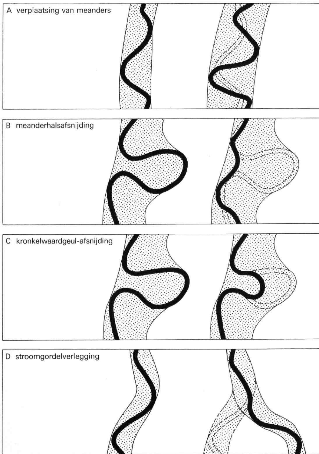
Fig. 5 Verschillende wijzen van riviervlegging.
