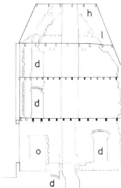
Afb. 41 Geertestraat 26 en 28. De zijgevels van nr 28. Tek. Kees Terhorst. A: de westmuur. B: de oostmuur. s: stookplaats. r: rookkanaal. n: nis. v: venster (1e fase). d: doorgang (1e fase). o: doorgang (2e fase). l: vliegringvloer (1e fase). h: haanhout.
