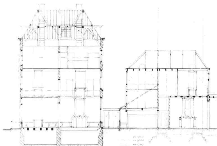
Afb. 71 Korte Nieuwstraat 6. Langsdoorsnede door het huis, naar het noorden gezien. Boven: de 17e-eeuwse opzet. Tek. A.F.E. Kipp. Onder: de huidige toestand. Tek. J.J. Jeehee en A. Warffemius (RDMZ), bewerkt en aangevuld door A.F.E. Kipp. Links het voorhuis, rechts het achterhuis met aanduiding van de verschillende groeifasen en gestippeld het westfront van de romaanse Pauluskerk, waar het oudste achterhuis tegen-aangebouwd was.
