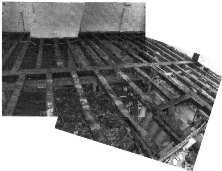
Afb. 32 Eligenstraat 39-45. De balklaag van nr 43 met vooraan rechts de vroegere trapraveling. Ook de zwaluwstaartverbinding van de raveelbalken van het rookkanaal met de moerbalk zijn duidelijk te zien. Op de achtergrond: de steunbeertjes van de tussenmuur.
