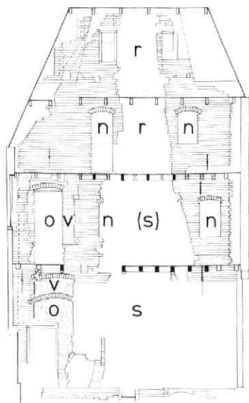
Afb. 41 Geertestraat 26 en 28. De zijgevels van nr 28. Tek. Kees Terhorst. A: de westmuur. B: de oostmuur. s: stookplaats. r: rookkanaal. n: nis. v: venster (1e fase). d: doorgang (1e fase). o: doorgang (2e fase). l: vliegringvloer (1e fase). h: haanhout.
