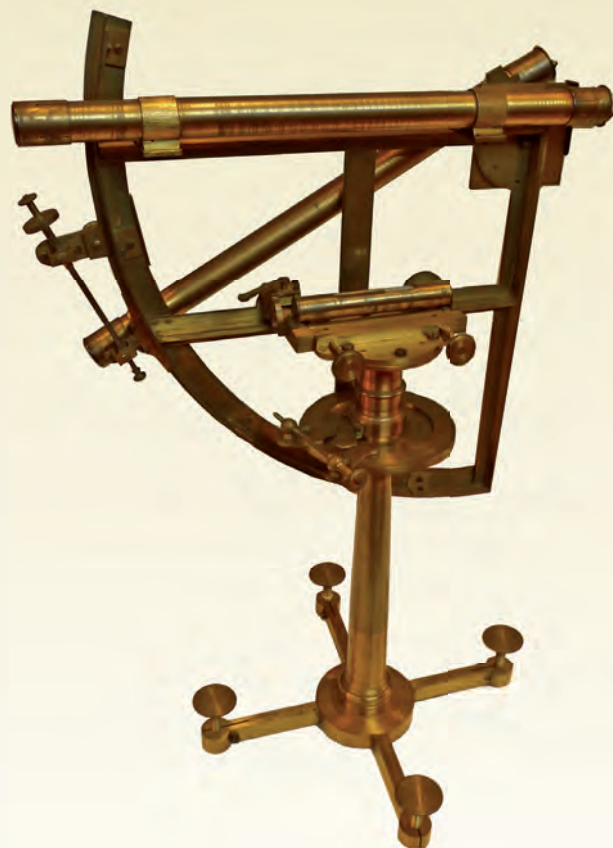
John Bird, astronomisch 12" quadrant vervaardigd voor Joan Gideon Loten 1771
