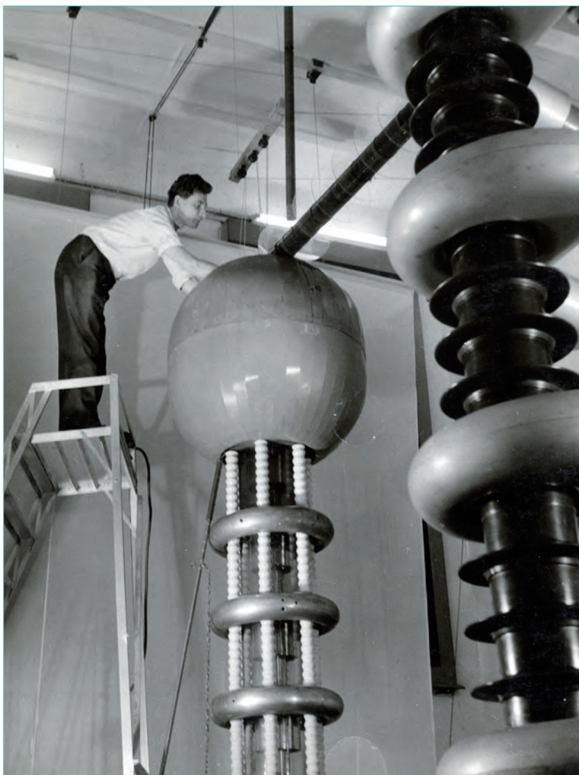
Hoogspanningsgenerator in het Fysisch Laboratorium (Bijlhouwerstraat), maart 1955.
