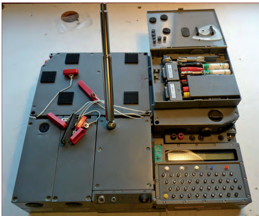
De FS-5000 was een door AEG Telefunken in 1985 ontwikkeld datacommunicatiesysteem voor het verzenden en ontvangen van gecodeerde boodschappen. Dit apparaat werd door verschillende stay behind-organisaties, waaronder de Nederlandse, gebruikt in de laatste operationele periode. In Nederland stond het systeem ook bekend onder de naam AZO-90 (Automatische ZendOntvanger 1990).
